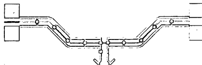
Fig. 5. Layout of LO balun
